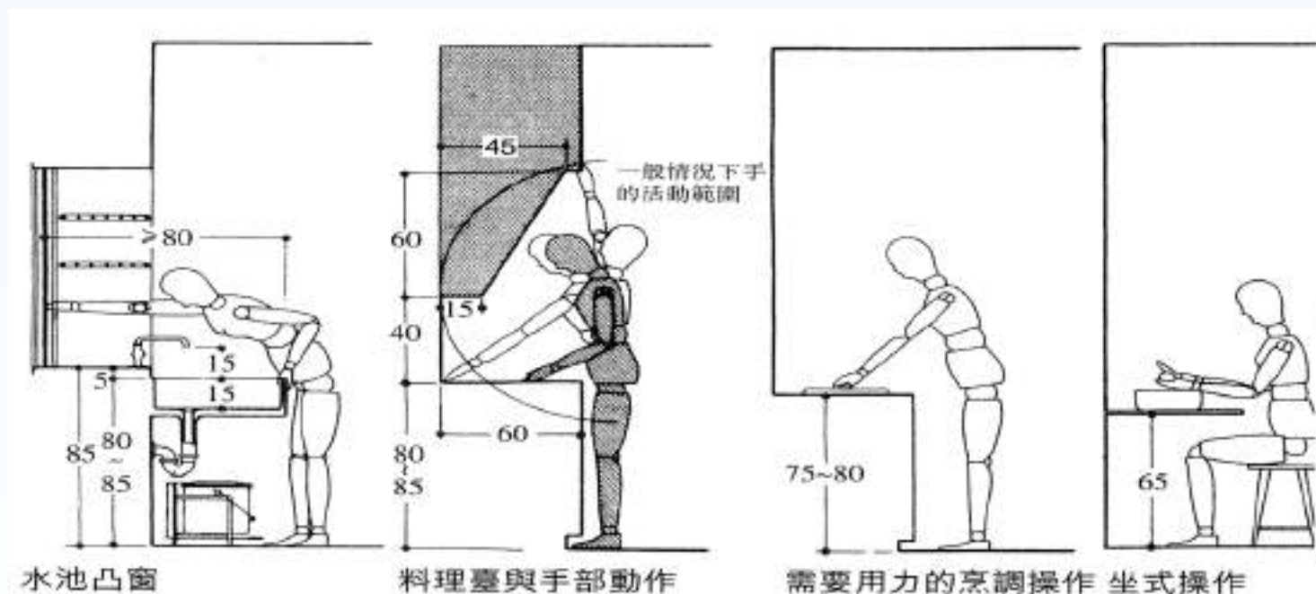
適當的廚房空間尺寸基準 (資料來源：日本建築學會，2002)
